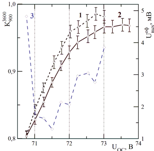
Рис.6. Зависимость усредненных значений амплитуд однофотоэлектронных сигналов МРРС S10931-100P (1) и S10931-050P (2) (правая шкала оси OY), и их обратных отношений (3) (левая шкала оси OY), от напряжения обратного смещения U_{OC} .
