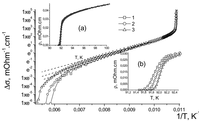
Рис. 1. Температурні залежності надлишкової провідності монокристалу YBa_2Cu_3O_{7-\delta} у координатах \ln\Delta\sigma - 1/T . Крива 1 отримана безпосередньо після зниження вмісту кисню, а криві 2 і 3 - після поетапного відпалювання експериментального зразка при кімнатних температурах протягом 20 годин і 5 днів, відповідно, без зміни вмісту кисню в об'ємі кристалу. Пунктирними лініями показані результати розрахунків за формулою (5). На вставці (а) показані температурні залежності електроопору \rho_{ab}(T) . На вставці (б) показані резистивні переходи в надпровідний стан.
